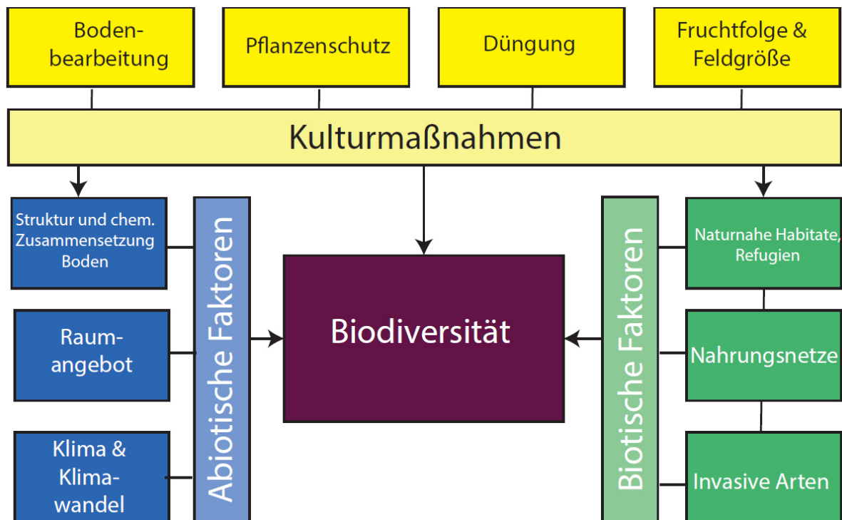
Abbildung 1: Wichtige Einflussfaktoren auf die Biodiversität der Agrarlandschaft
