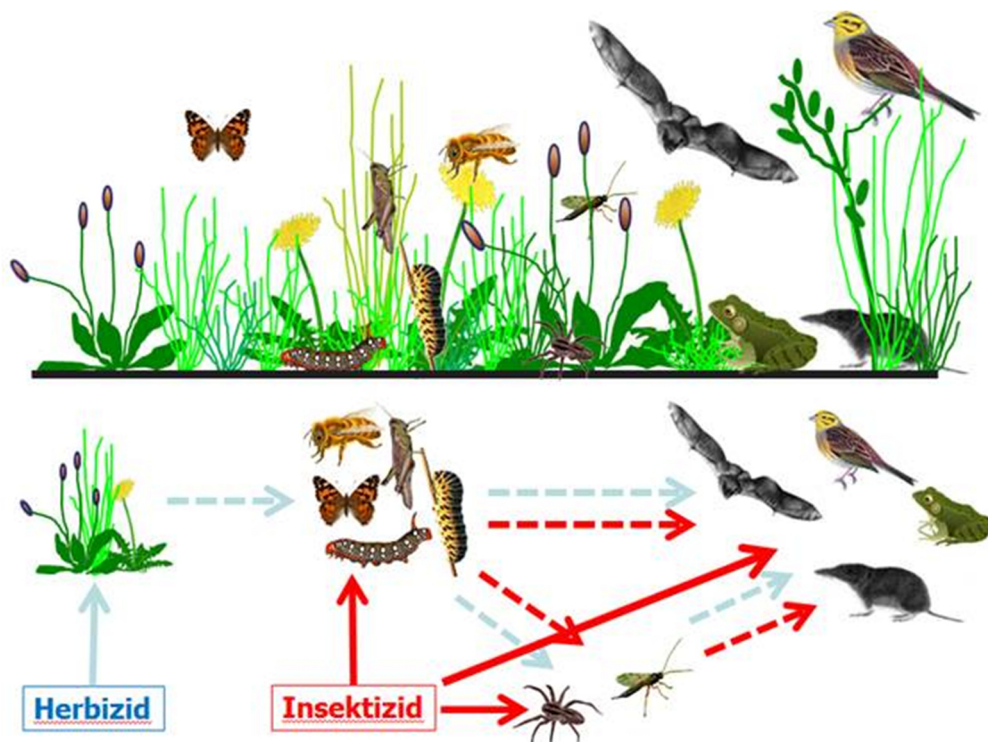
Abbildung 2. Nahrungsnetz in Feldrändern. Direkte negative Wirkungen (durchgezogene Pfeile) und indirekte Wirkungen (gestrichelte Pfeile) von Herbiziden (blau) und Insektiziden (rot). 50
